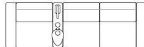
1B + SB CONSOLE + 1B (BRAÇO: 15 OU 25CM) (FORM. CONSOLE: RETO OU ANGULAR) (COMP. CONSOLE: 25 OU 40CM) (LAD. CONSOLE: DIREITO OU ESQUERDO) ASS 0,80 x 1,12 m | 31 4/8 in x 44 1/8 in 3 0,90 x 1,12 m | 35 3/8 in x 44 1/8 in 3 1,10 x 1,12 m | 43 2/8 in x 44 1/8 in 3
